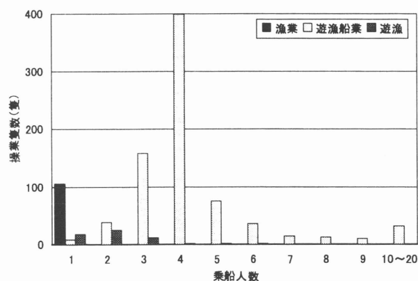
図10-6 船別乗船人数
