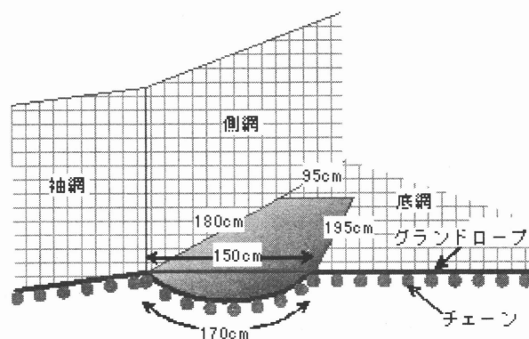
図2 カイト模式図
