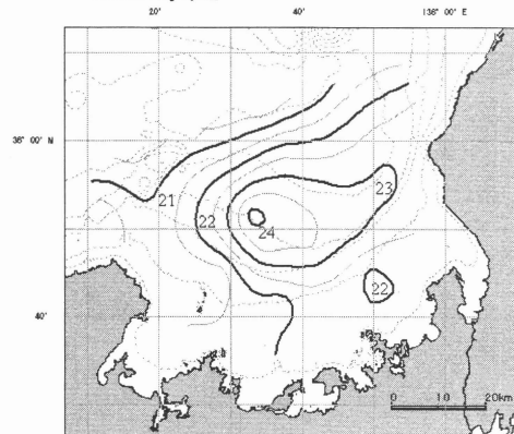
100m 水温
