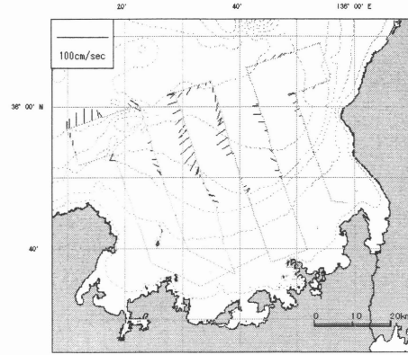
図 2-3 若狭湾海域水温水平分布および潮流（平成 20 年 8 月 6 日～7 日）
