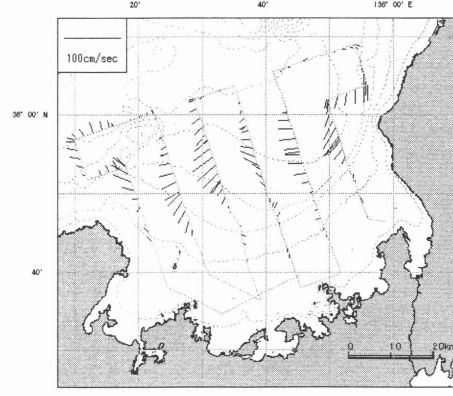
150m層潮流
