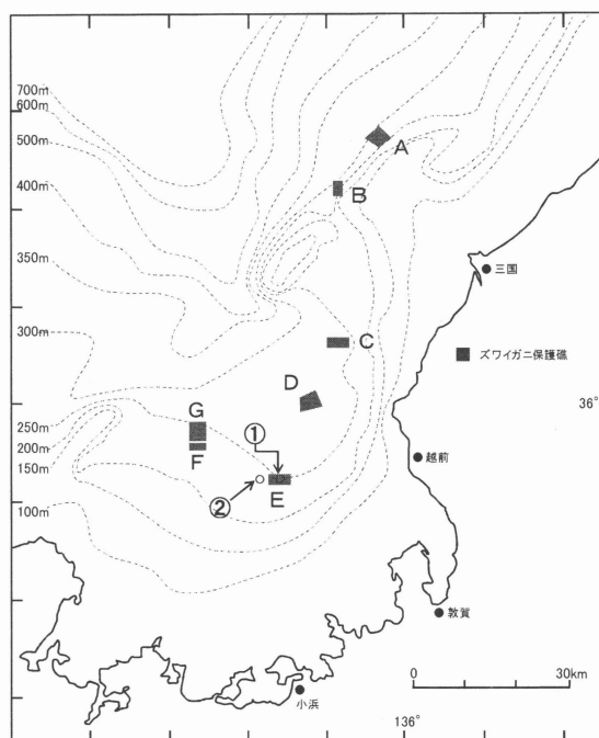
図1 調査海域図
