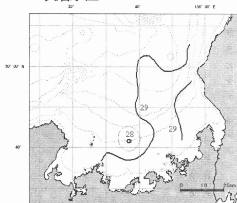
50m 水温
