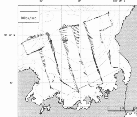
50m層潮流
