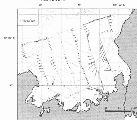
100m層潮流
