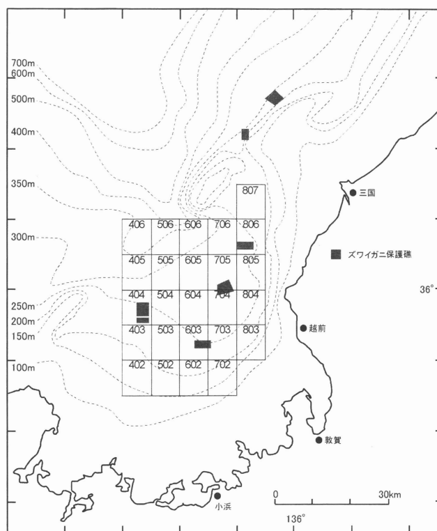
図 1 調査海域図
