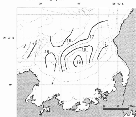
150m 水温
