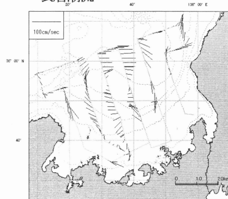
50m層潮流
